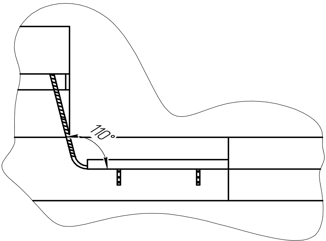
Рамка-суппорт на 6 модулей, PDA-3DN
