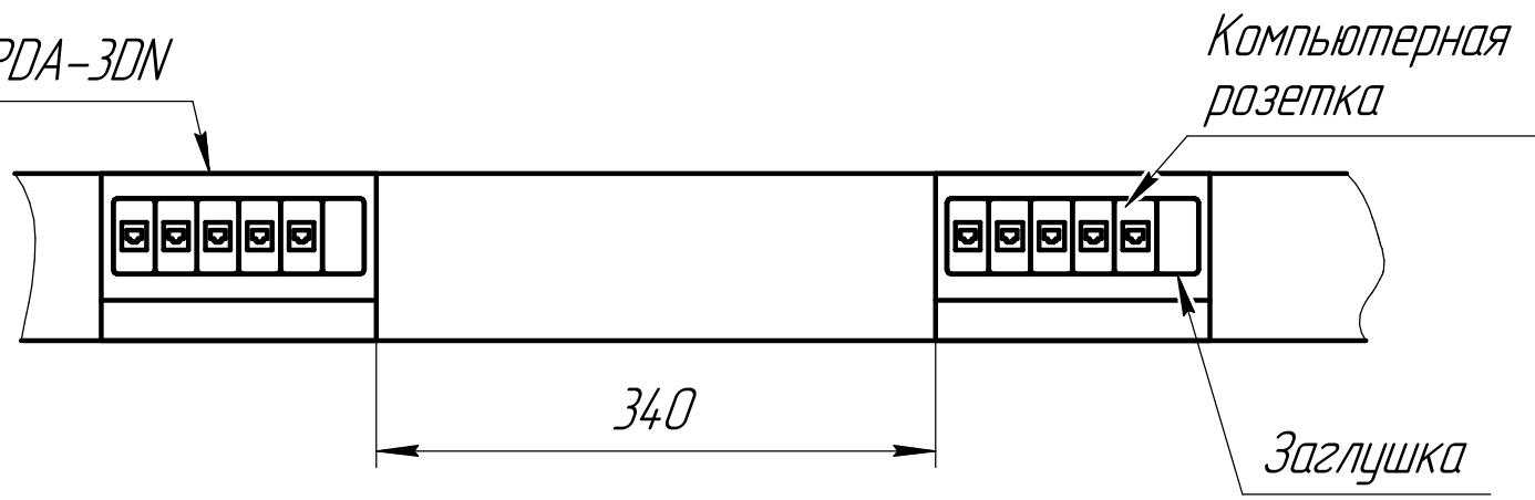
Расположение рамок-суппорт на кабель-канале
