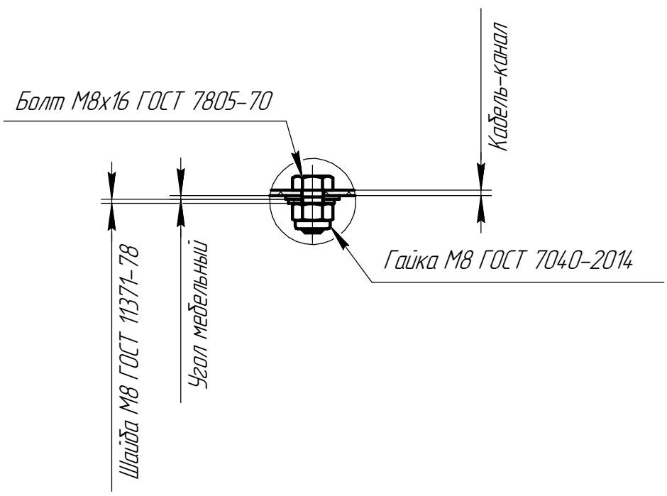
Крепление кабель-канала к медельному уголку
