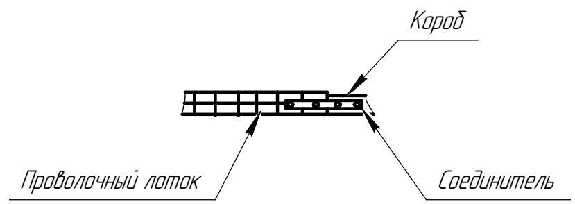
Схема крепления короба к лотку
